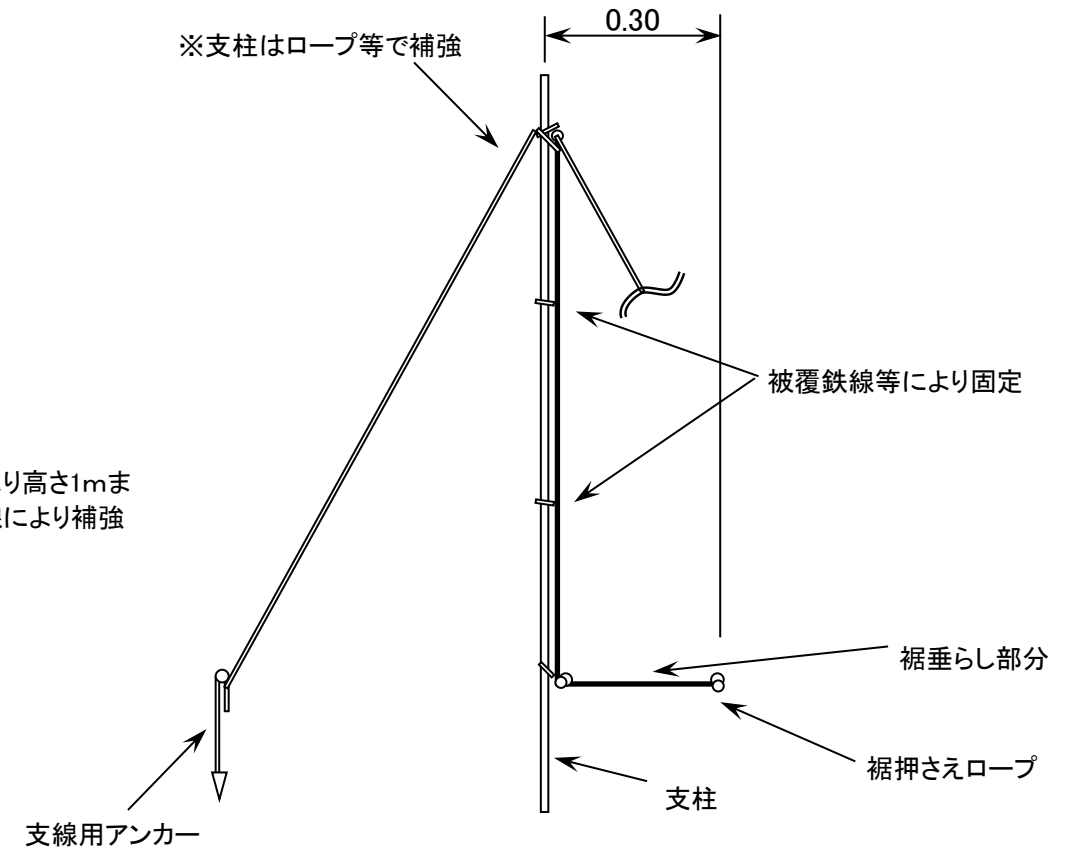
側 面 図
