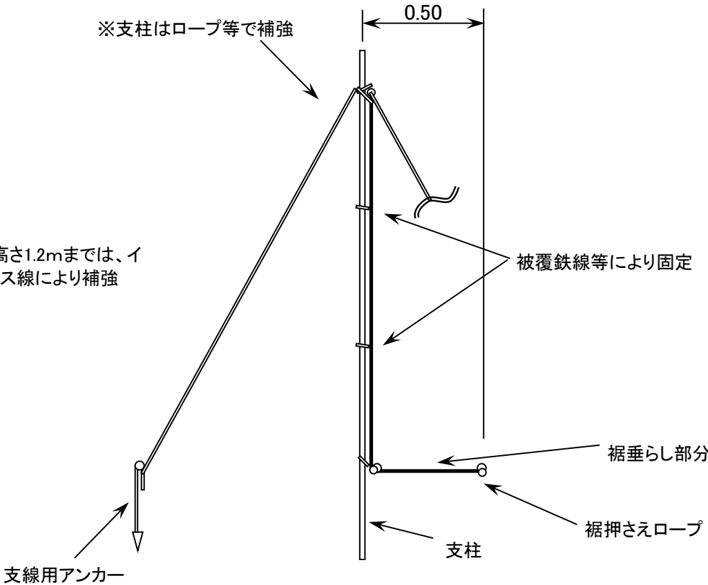
側面図
